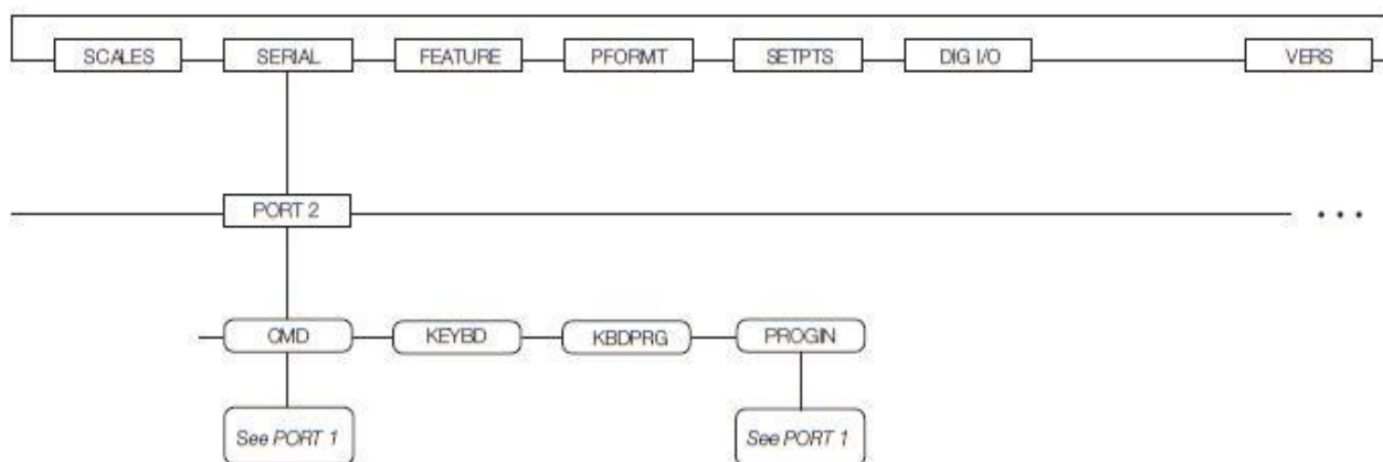
图:3-10. 串口子菜单, 串口2(带串行口选项)
