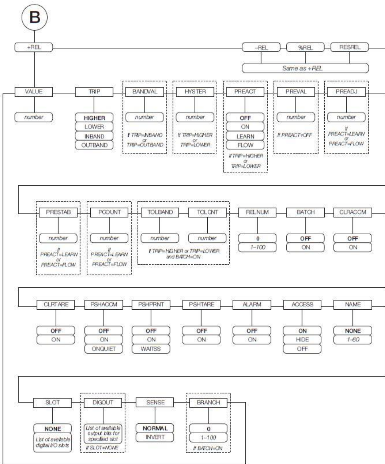
图9-3.+REL、-REL、%REL、SRESREL设定点参数
