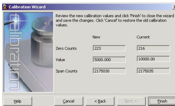
图:4-10. iRev 4 校准值界面
