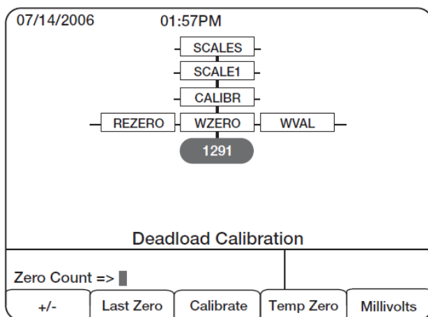
图4-2. WZERO(零点)校准界面
